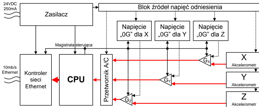
Rysunek 8. Architektura akcelerometru ADXL001-70.
