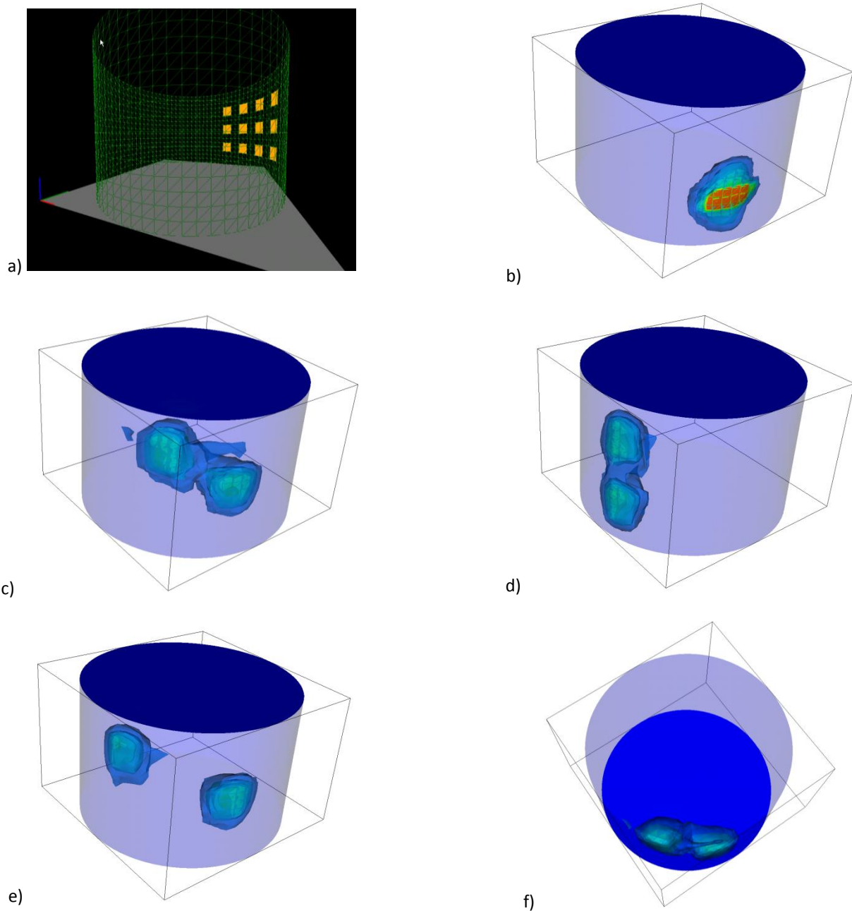
Rysunek 21. Wizualizacja map czułości dla wybranych elektrod czujnika ECT, a) rozmieszczenie elektrod, b) mapa czułości między przyległymi elektrodami z dwóch poziomów, c) mapa czułości między naprzeminoległymi elektrodami z dwóch poziomów, d) mapa czułości między
