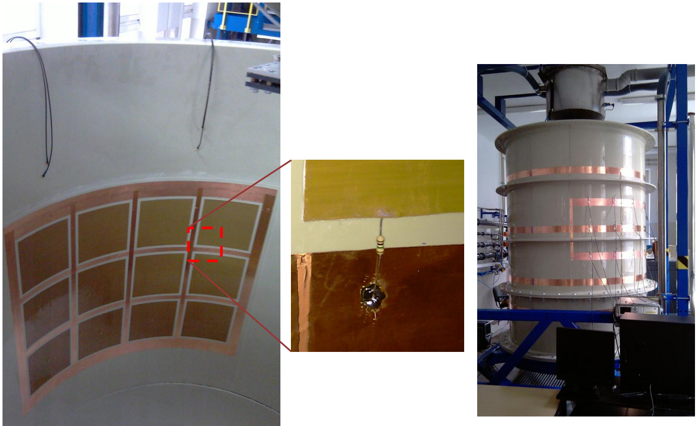
Rysunek 22. Zdjęcie czujnika pomiarowego 3D ECT, a) widok czujnika 3D ECT od strony wnętrza silosu, b) widok ekranów zewnętrznych czujnika 3D ECT
