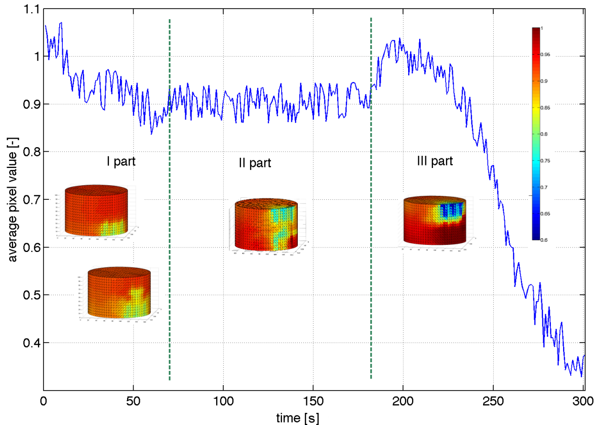
Rysunek Wykres zmian średniej wartości koncentracji materiału w obszarze czułości pomiarowej czujnika ECT z naniesionymi zrekonstruowanymi obrazami dla trzech głównych etapów opróżniania silosu.
