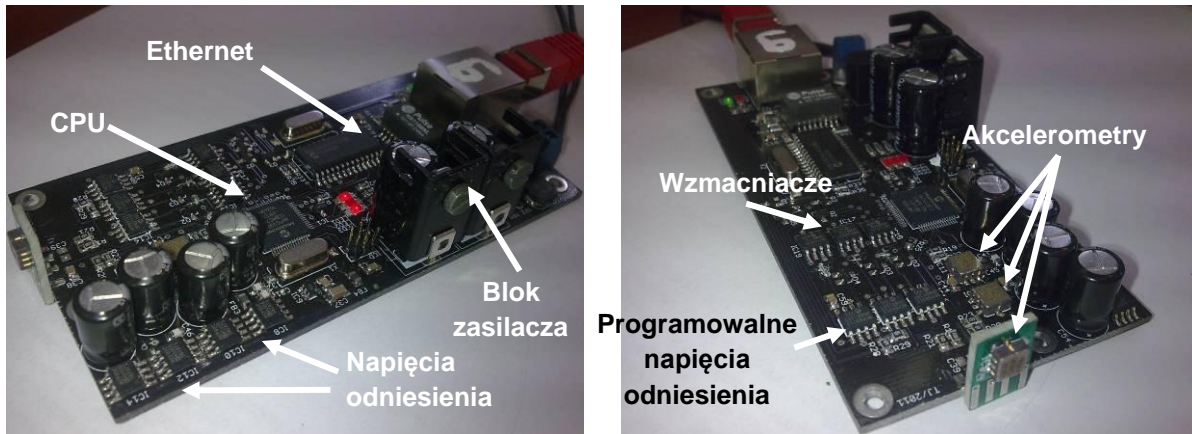
Rysunek 9. Płytki PCB z zamontowanym trójosiowym układem akcelerometrów
