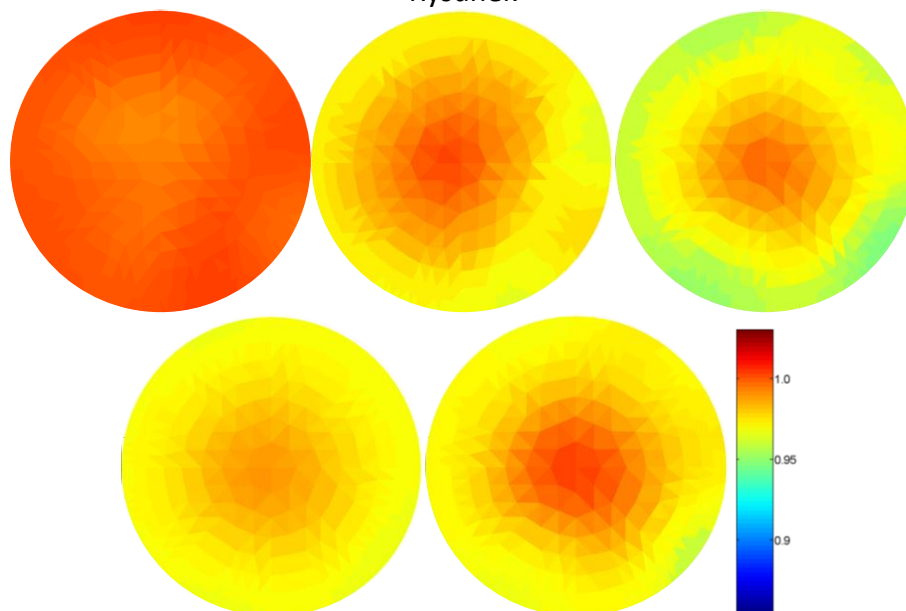
Rysunek Przykładowe zrekonstruowane obrazy metodą G-N dla chwil czasu: 20 s, 30s, 40s, 50, 60 s.
