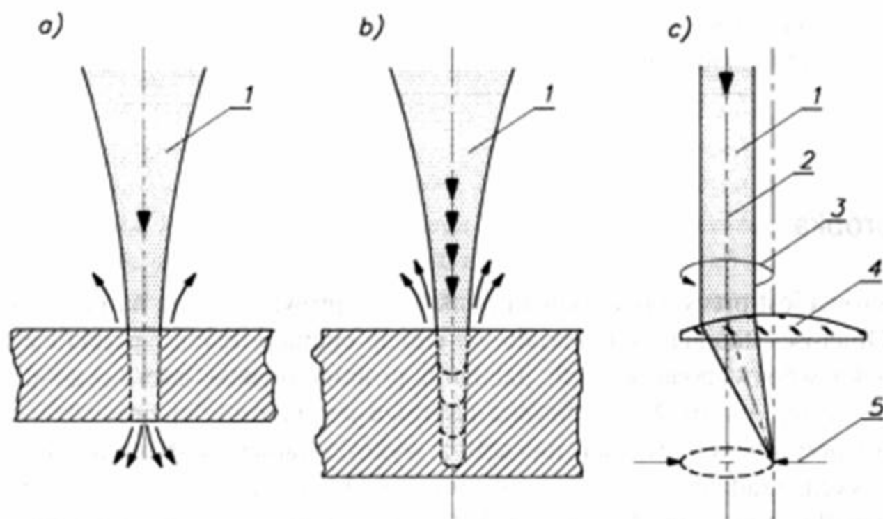
Rys. 11.17. Drażenie laserowe, wg [696]: a) perforacyjnej; b) perkusyjnej; c) trepanacyjnej 1 – wiązka laserowa, 2 – oś drążonego otworu, 3 – rotacja soczewki wokół osi otworu, 4 – soczewka, 5 – średnica drążonego otworu
