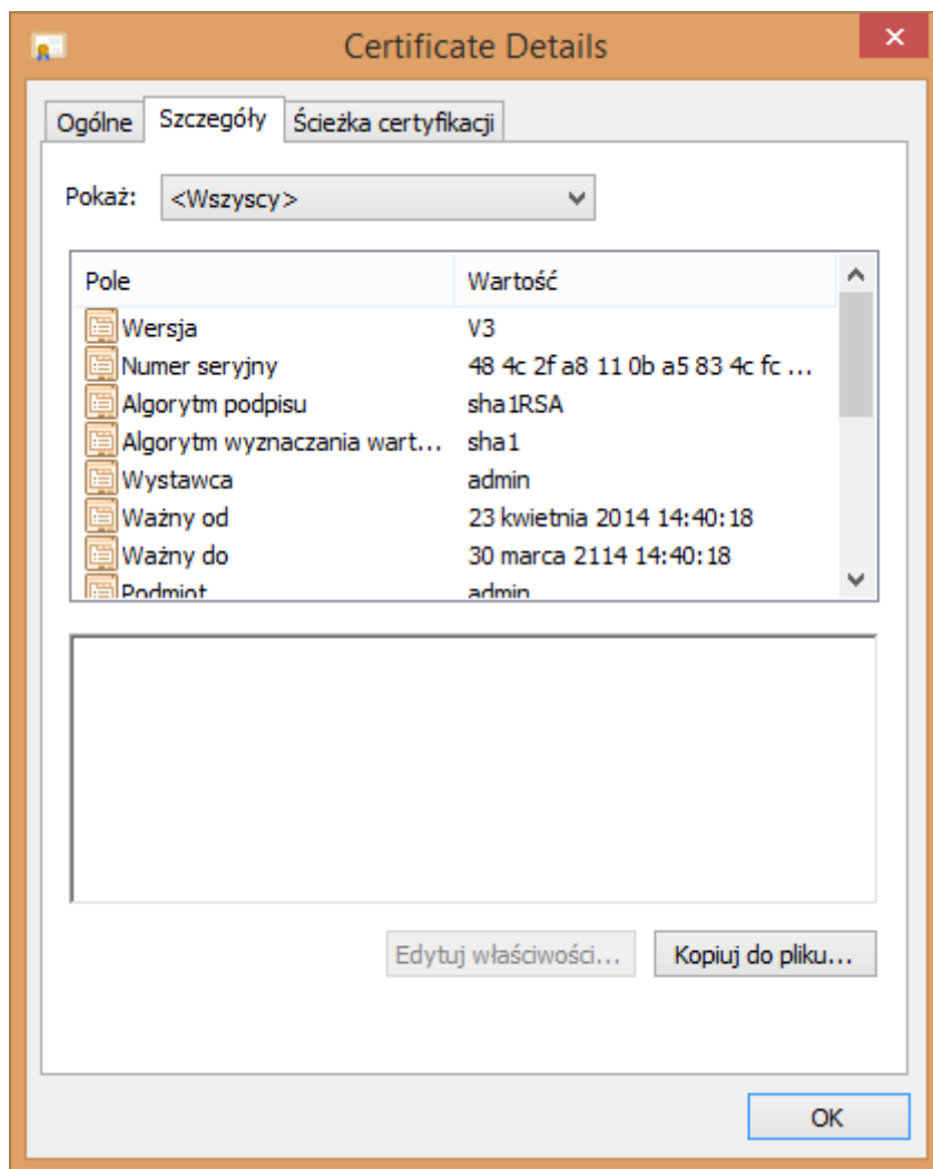
Rys. 8 Okno certyfikatu użytkownika
